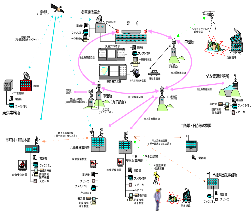
福岡県防災・行政情報通信ネットワーク(ふくおかハイパーネット)概念図
