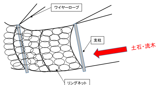
【アンカーネット式構造物イメージ図】
