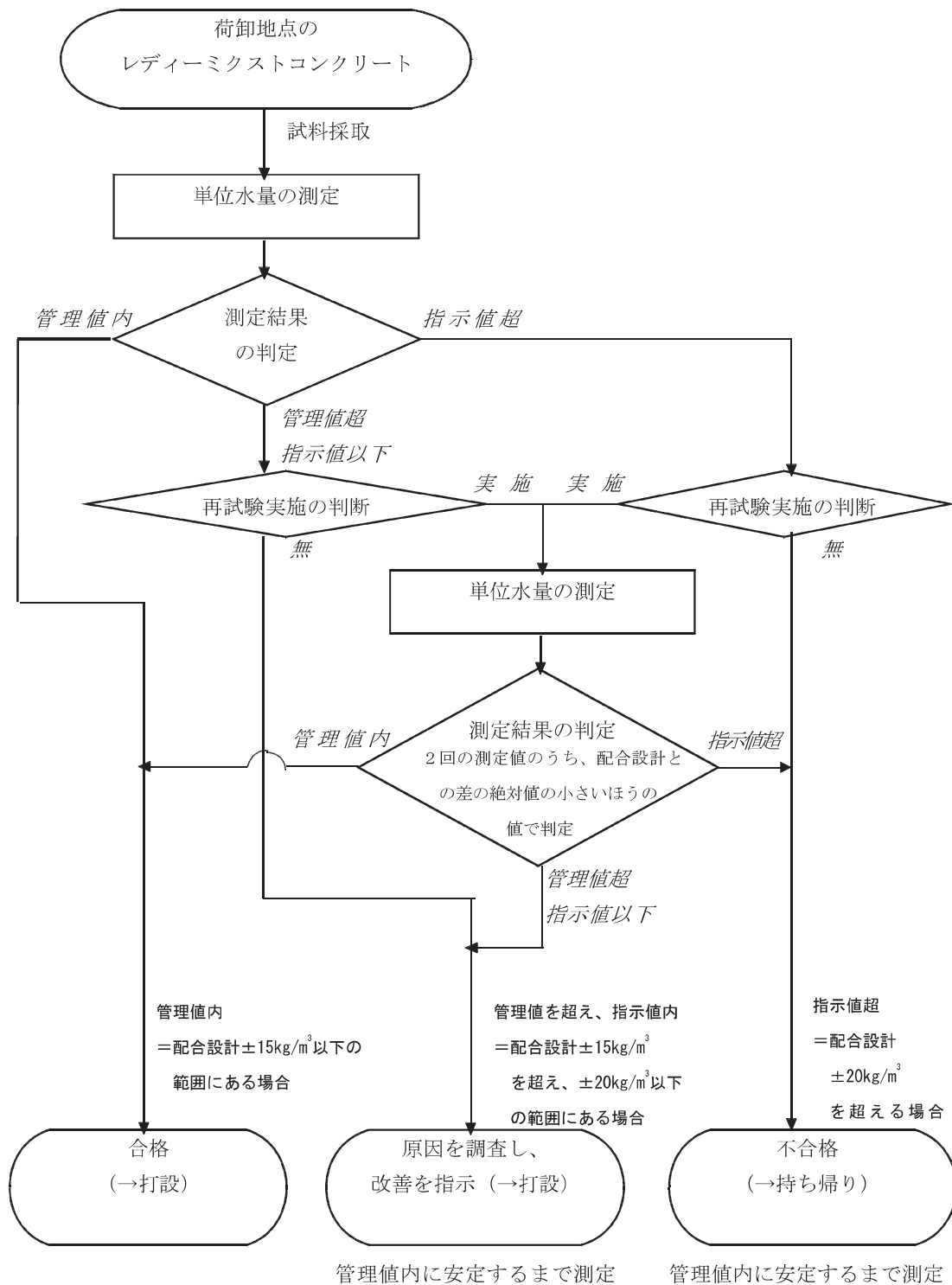
レディーミクストコンクリートの単位水量測定の実行フロー図
