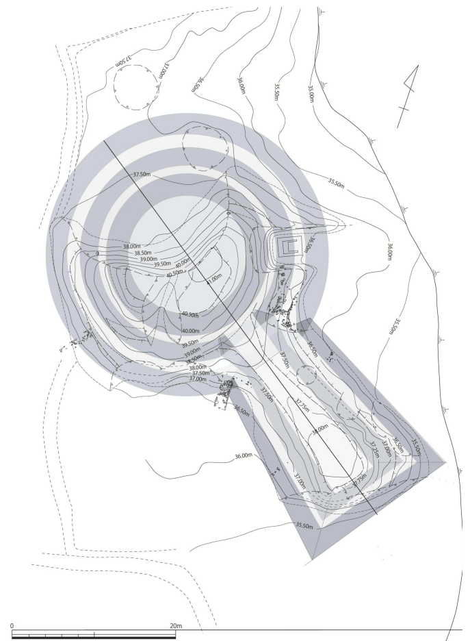
图3 西方古墳復元実測图
