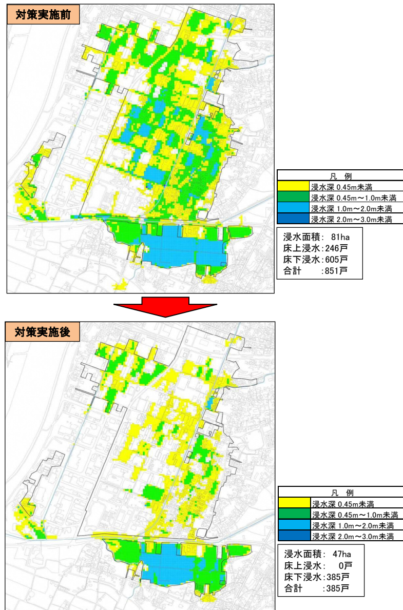
図 4-41 対策実施の効果(浸水深)
