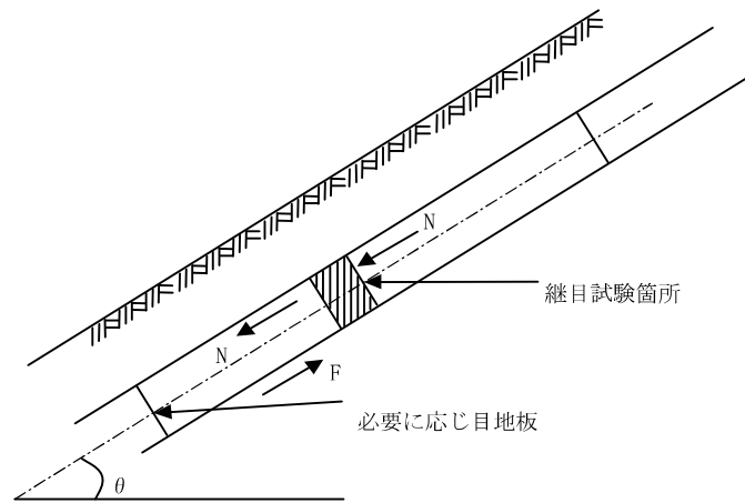
図－２ 継目試験箇所及び力
