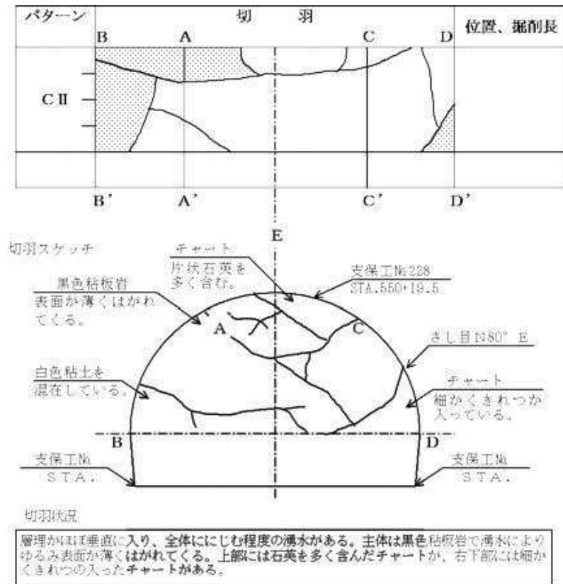
図ー1 切羽観察調査の様式と記載例
