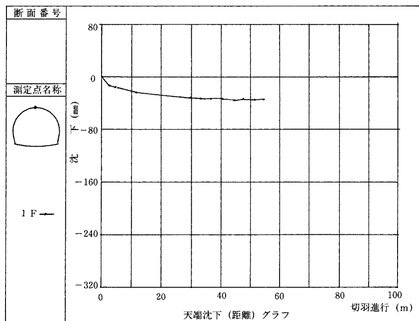
図－４ 天端沈下変化図(例)
