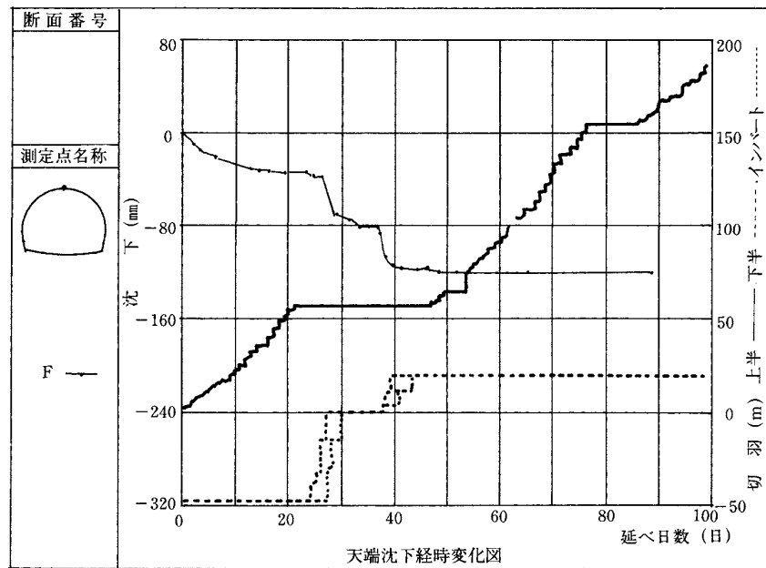
図－３ 天端沈下経時変化図(例)
