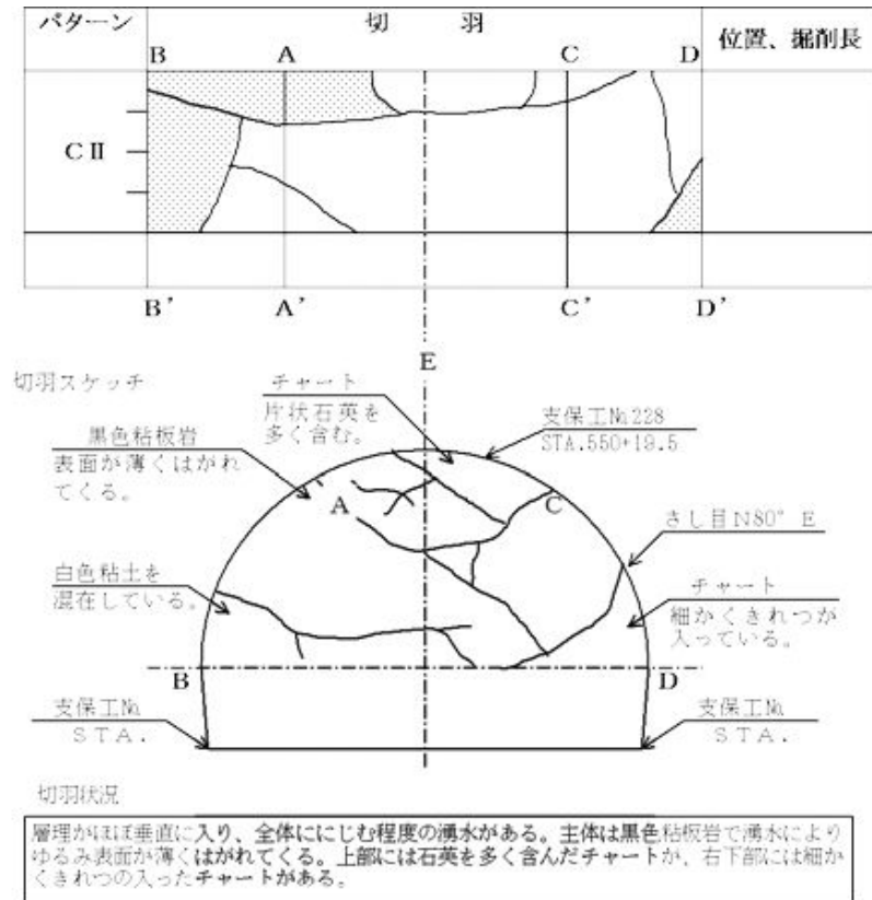
図ー1 切羽観察調査の様式と記載例
