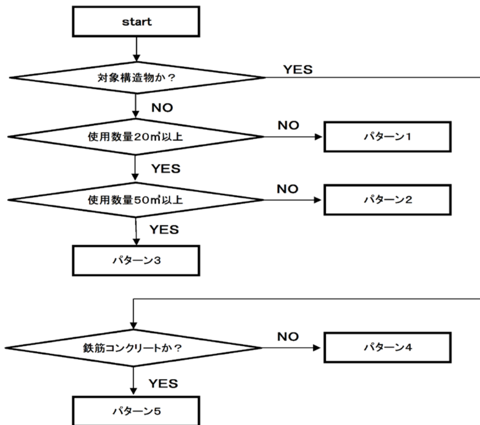
コンクリート圧縮強度の品質管理試験フロー
