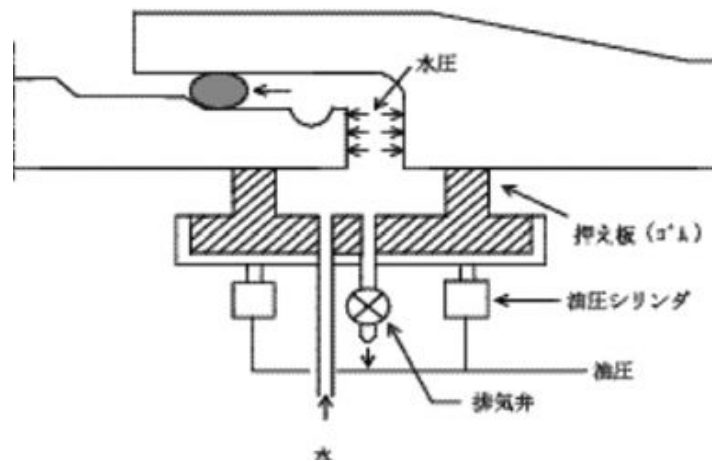
図ー３ テストバンドの機構の概略
