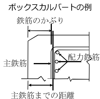
図 3-9-1 鉄筋のかぶり
