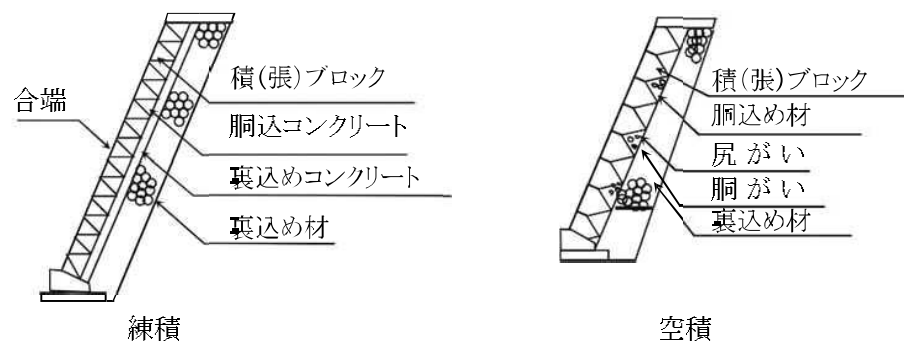
図 3-3-4 コンクリートブロック工
