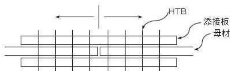
図 3-3-1 ボルト締付け順序
