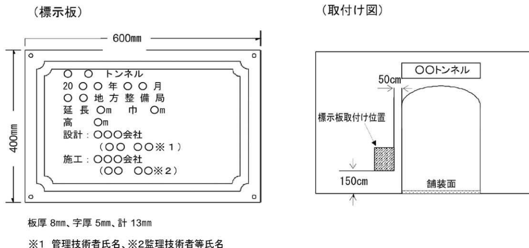
図 6-7-2 標示板の設置イメージ図
