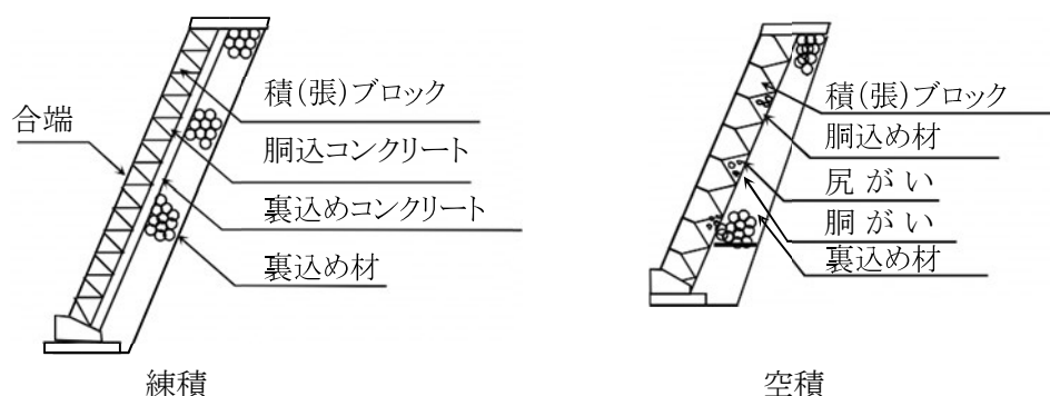
図 3-2-5 コンクリートブロック工
