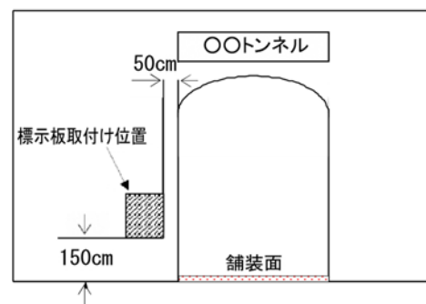
(取付け図)
