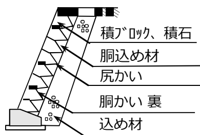
空積
