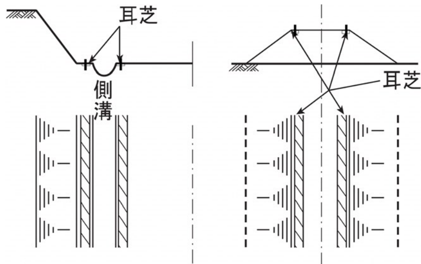
図 3-3-6 耳芝
