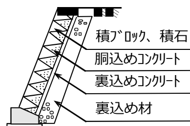
練積
