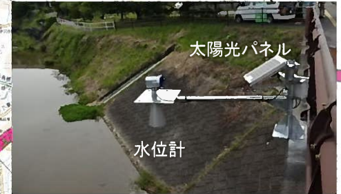
危機管理型水位計設置(例)
