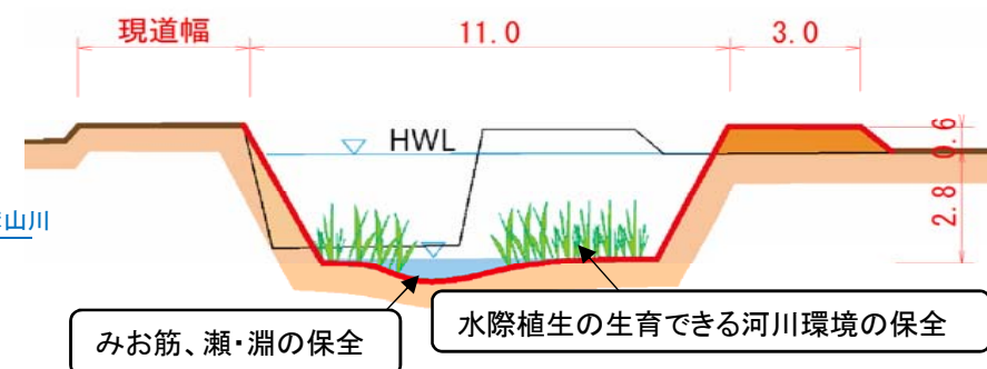
【計画標準横断面図】
