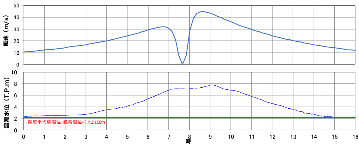
図-15 代表コースでの風速・潮位の時間変化 (3)
