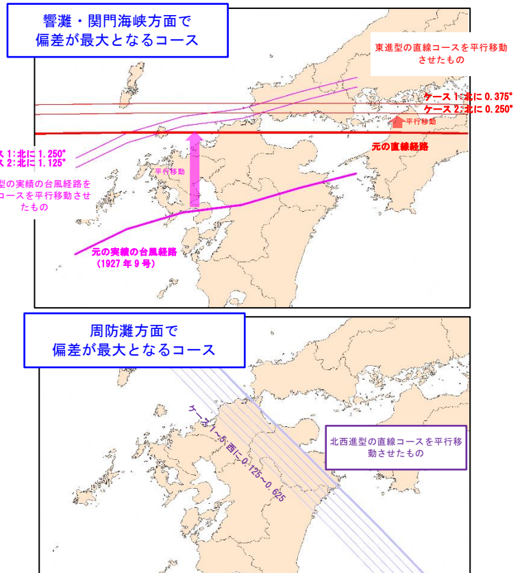
図-10 豊前豊後沿岸各地点で偏差が最大となる台風のコース(上：響灘・関門海峡、下：周防灘)
