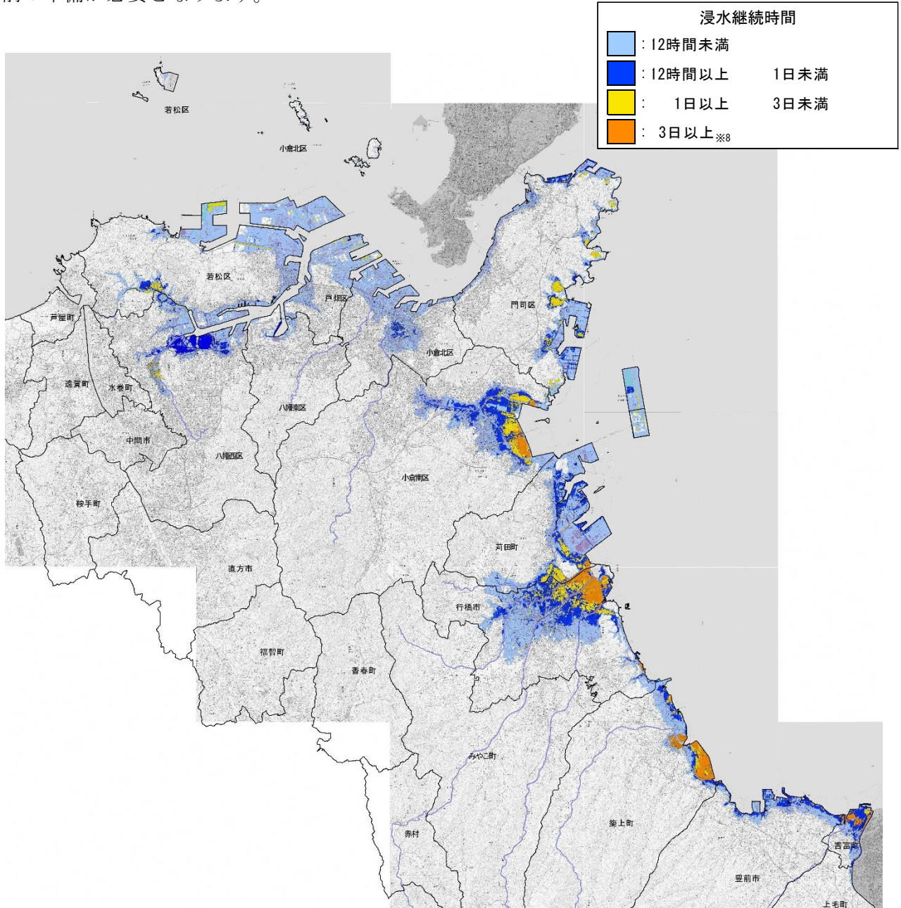
図－16 豊前豊後沿岸での最大規模の高潮に対する浸水継続時間
