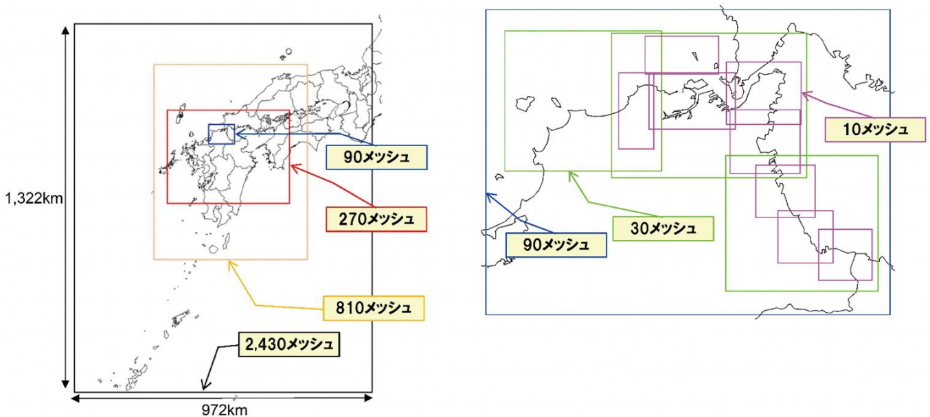
図－1 2 計算領域及び計算格子間隔
