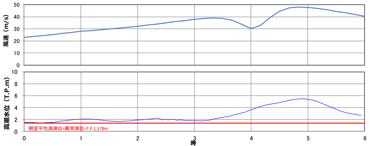
図-15 代表コースでの風速・潮位の時間変化（1）
