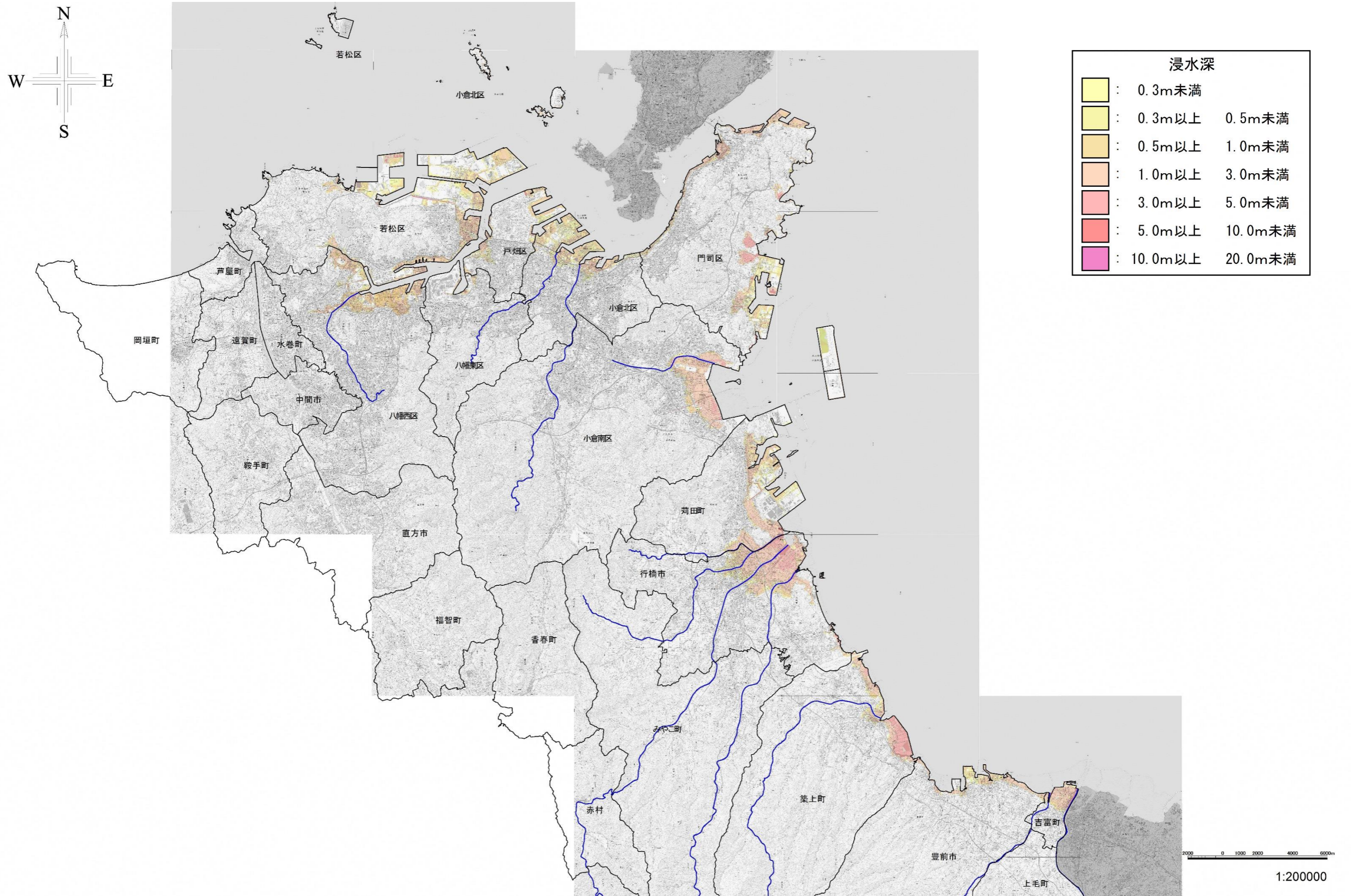
図-5 福岡県豊前豊後沿岸での北東進型 (930 hPa) の最大浸水深分布
