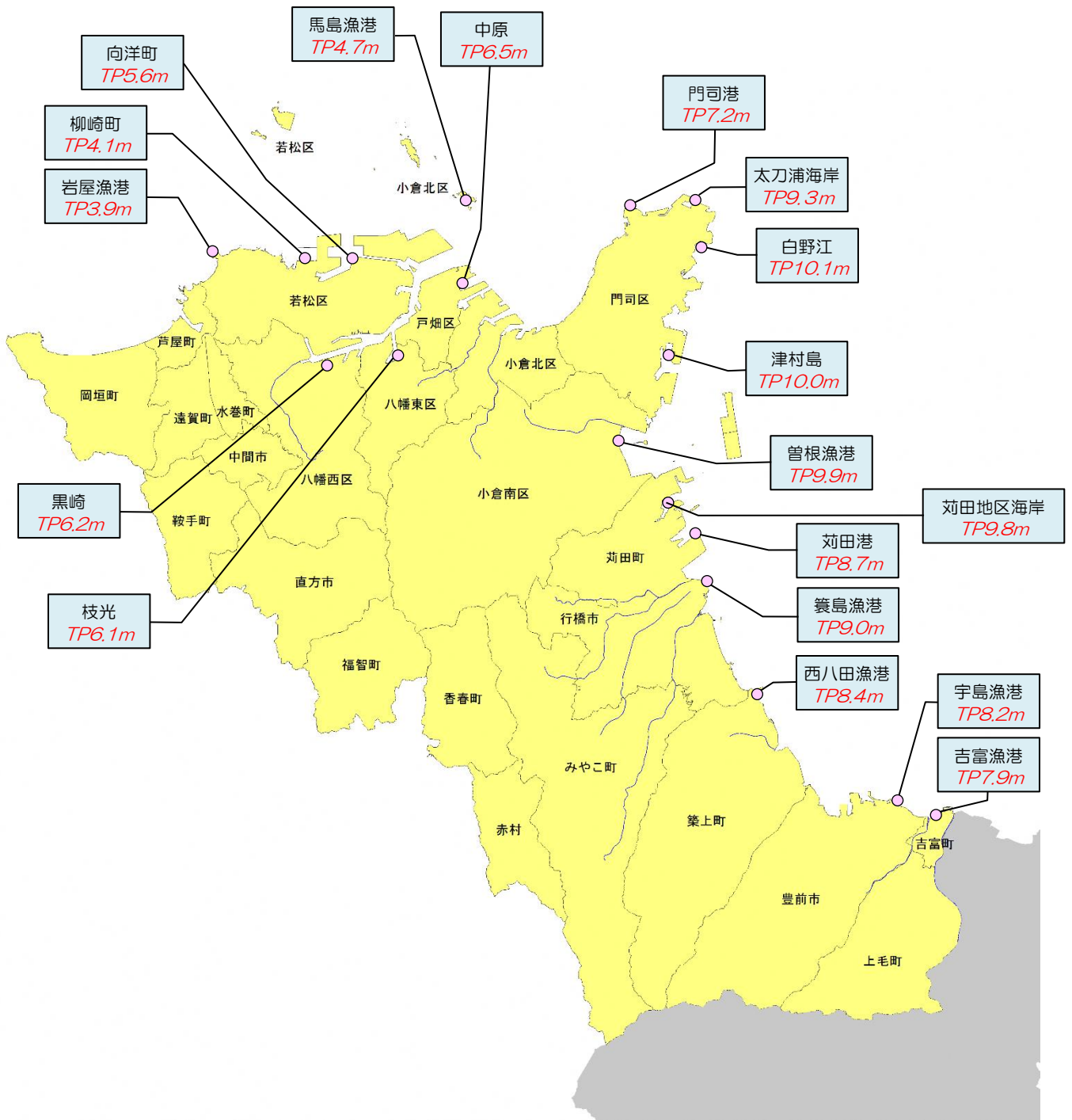
図－6 各市町の代表地点における高潮水位
