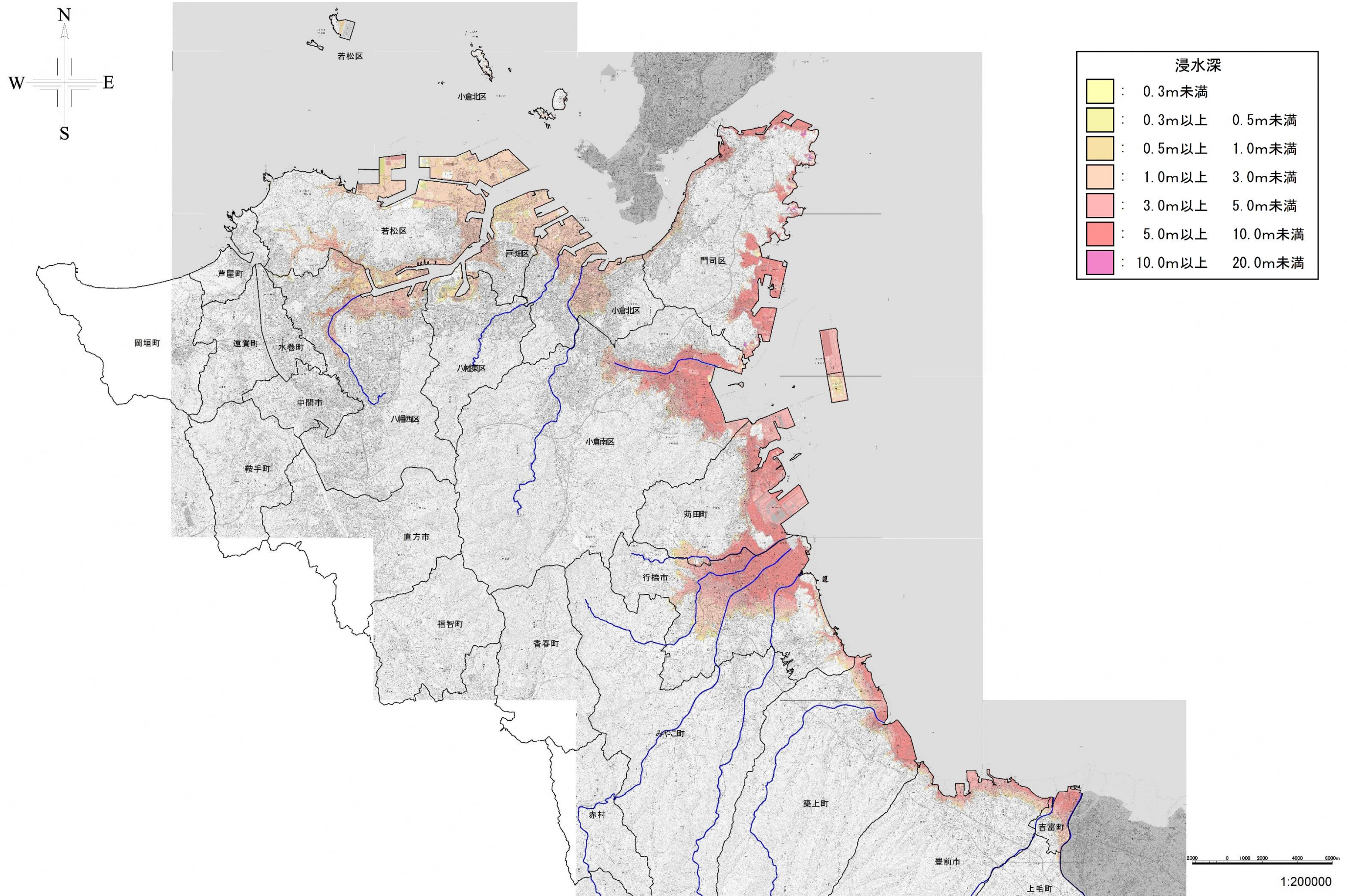
図-13 福岡県豊前豊後沿岸での最大規模高潮による最大浸水深分布
