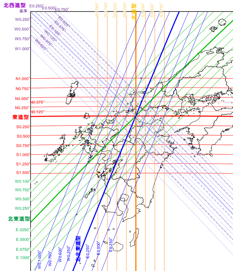
図-3 各方向を直線化したものを平行移動させた想定台風のコース
