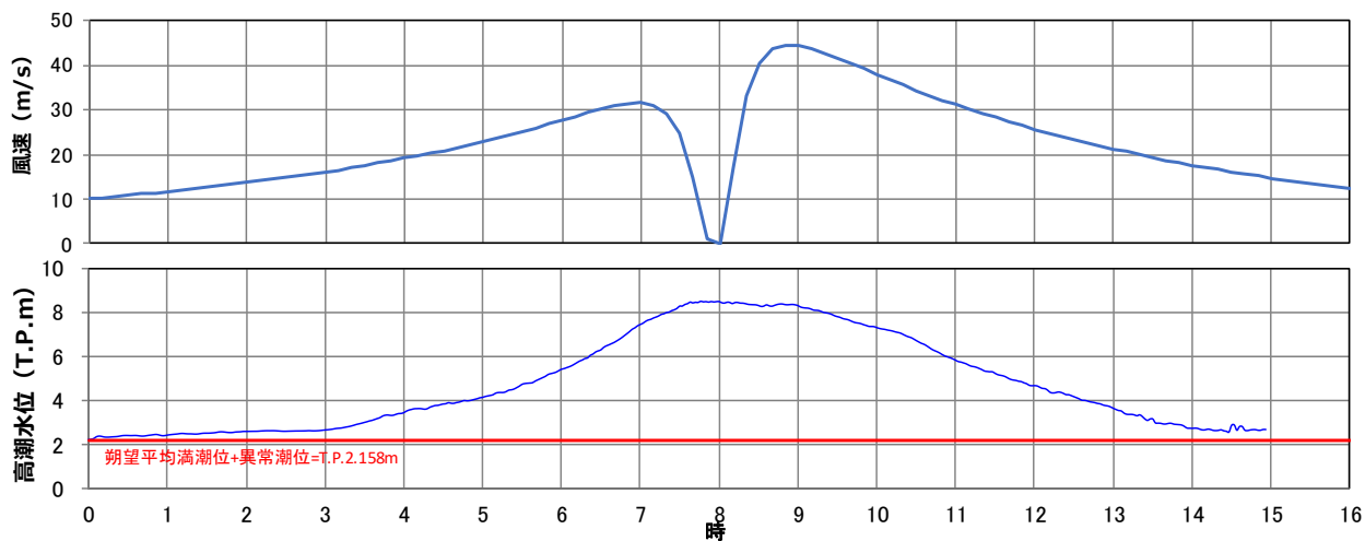
図-15 代表コースでの風速・潮位の時間変化（2）
