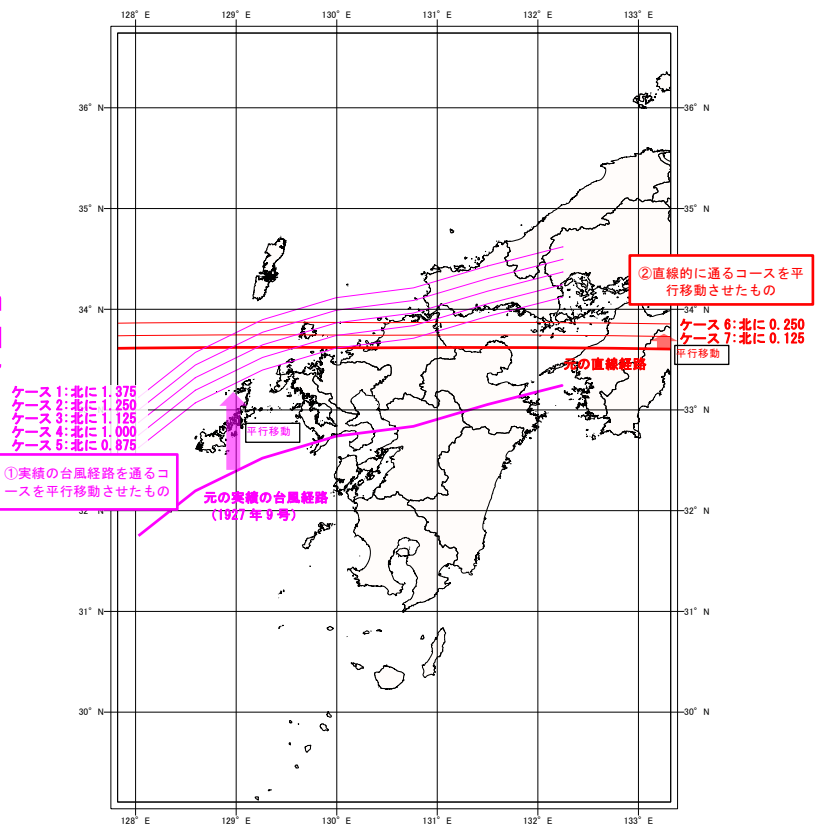
図-9 玄界灘沿岸各地点で偏差が 最大となる台風のコース
