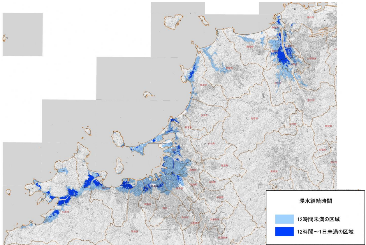
図－15 玄界灘沿岸での最大規模の高潮に対する浸水継続時間
