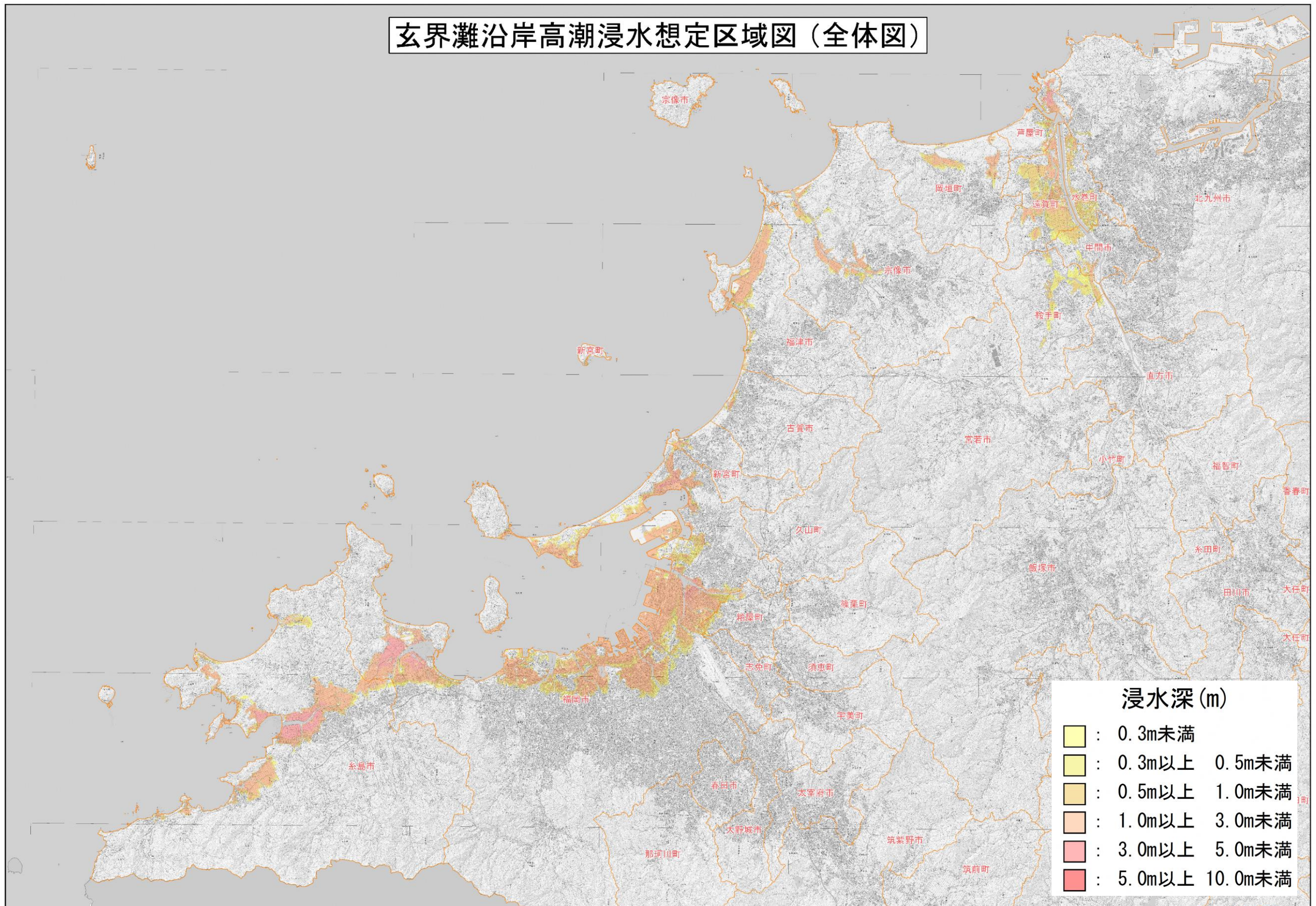
図-17 福岡県玄界灘沿岸での北東進型（930 hPa）の最大浸水深分布
