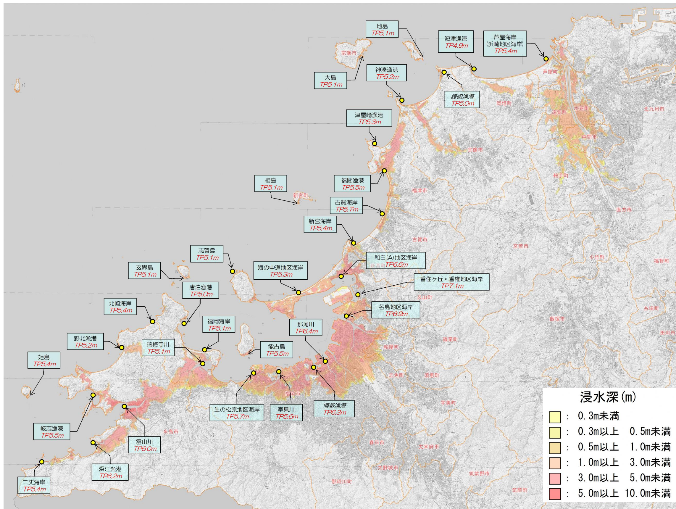
図-12 福岡県玄界灘沿岸での最大規模高潮による最大浸水深分布と、代表地点での最大高潮水位
