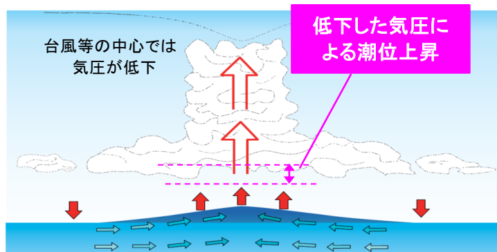
図-3 吸い上げ効果
