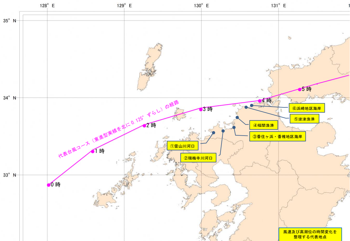
図-13 代表コースの台風経路
