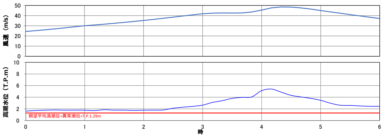
図-14 代表コースでの風速・潮位の時間変化 (2)
