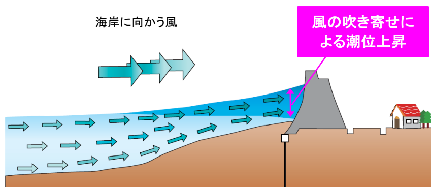
図-4 吹き寄せ効果
