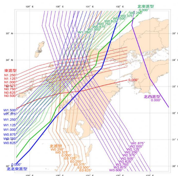
図－1 実績コースを平行移動させた想定台風のコース
