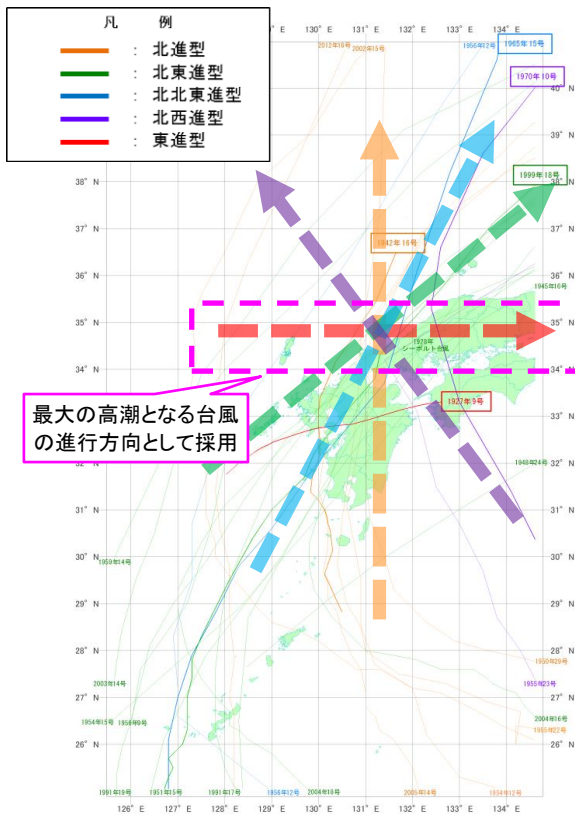
図-8 玄界灘にとって高潮の危険がある 台風の進行方向
