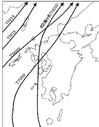
有明海に高潮被害が発生した時の台風経路
