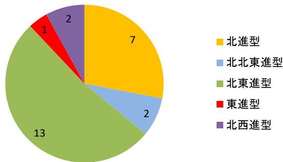
図-16 玄界灘に来襲した台風コースの割合
