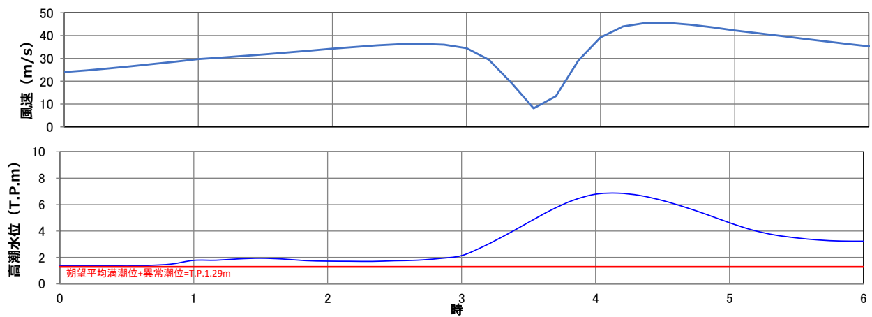
図-14 代表コースでの風速・潮位の時間変化 (1)
