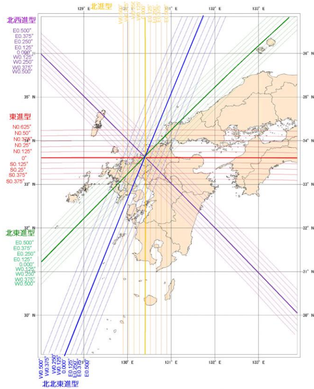
図-3 各方向を直線化したものを平行移動させた想定台風のコース
