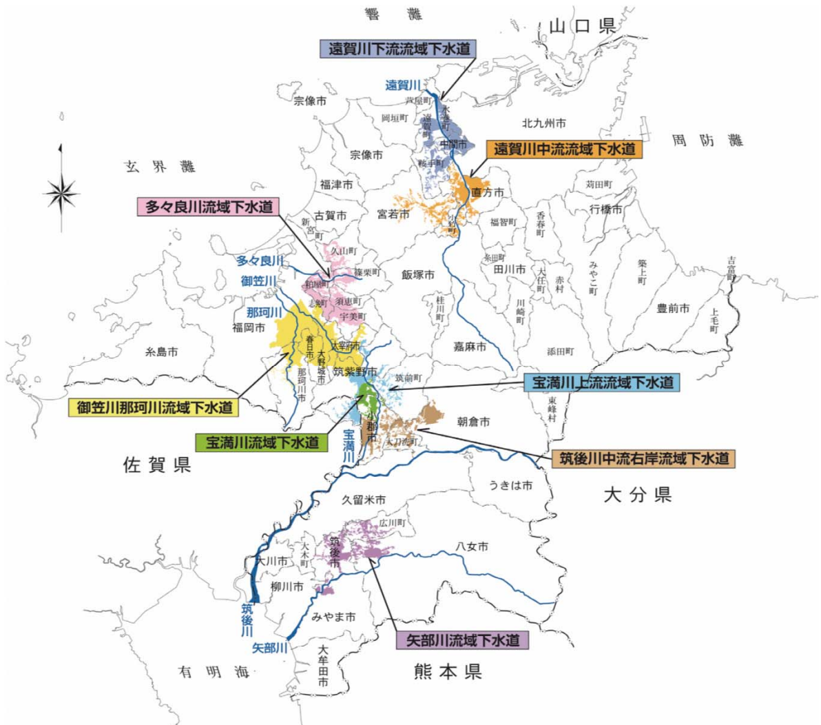
福岡県流域下水道概要図
