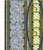
コンクリート増打ち
