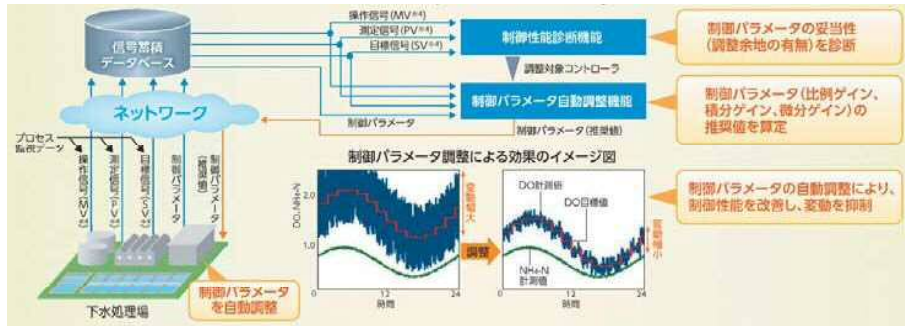
図III-25 制御性能改善技術の概要
