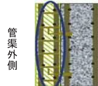
管外面へのコンクリート増打ち
