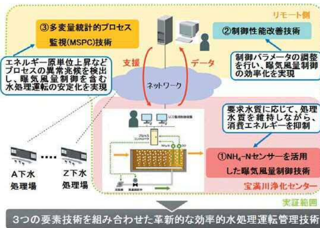
図Ⅲ-23 実証技術の概要
