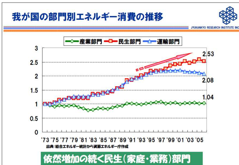
【資料1】 我が国の部門別エネルギー消費 出典：(株)住環境計画研究所 中上英俊会長，第3回研究会講演資料
