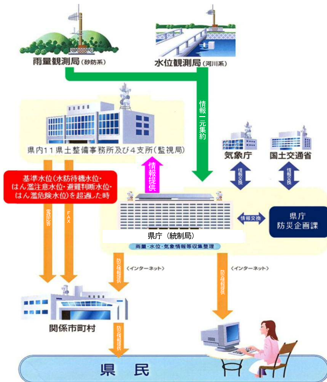
福岡県総合防災情報システムネットワーク図
