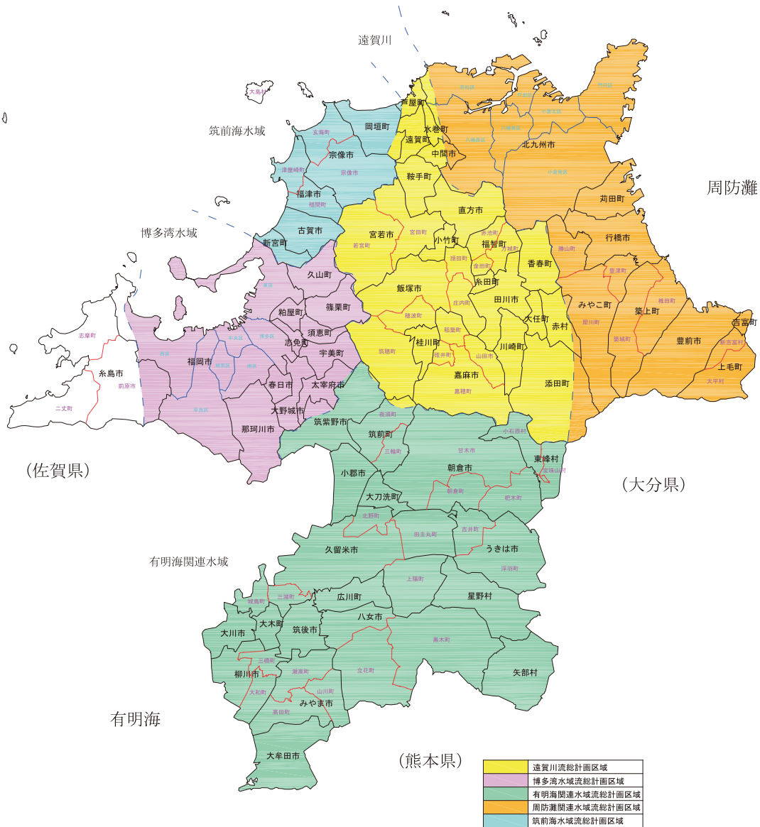
図 V-4 流域別下水道整備総合計画調査区域図
