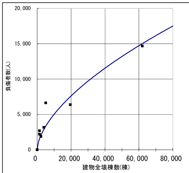
図 3.2-2 負傷者数と建物全壊棟数との関係
