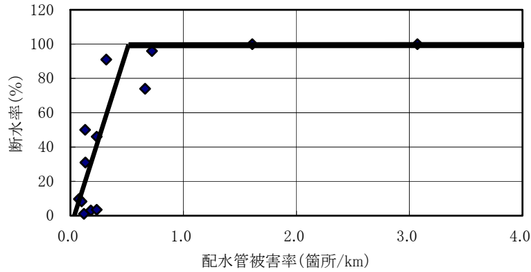
図 3.2-3 上水道管の被害率と断水率の関係
