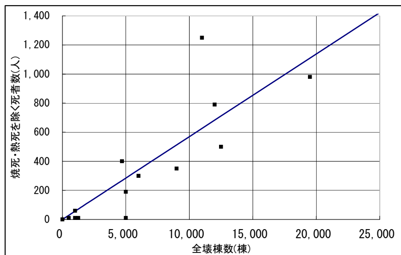
図 3.2-1 死者数と建物全壊棟数の関係 (池田・中林 1996)
