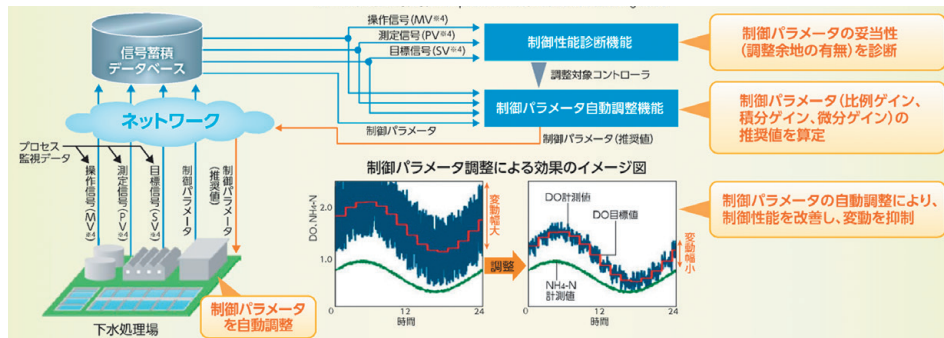
図Ⅲ-25 制御性能改善技術の概要
