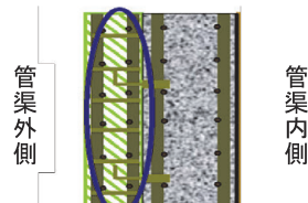
管外面へのコンクリート増打ち
