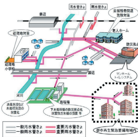
下水道総合地震対策事業のイメージ
