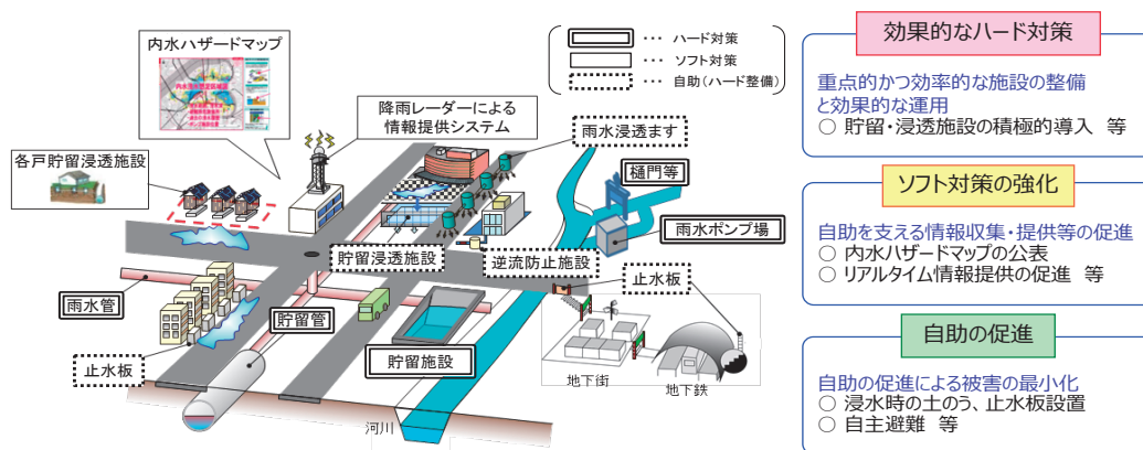
下水道浸水被害軽減総合事業のイメージ
