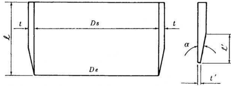
図 3-1 サンプルチューブ
