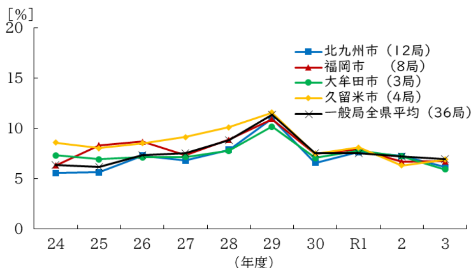
光化学オキシダントの経年変化（一般環境大気測定局） ～昼間0.06ppm（環境基準）を越えた時間数割合～
