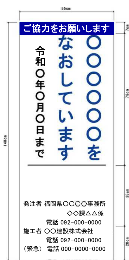
(様式2) 工事説明看板 (例：道路補修工事)
