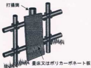
図8. 畳床(例)
